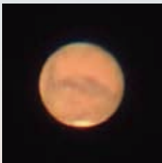
▲(図1)美星天文台で撮影した火星
