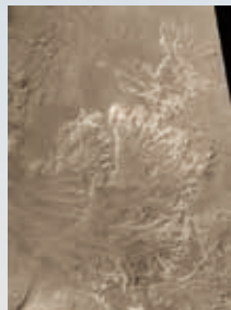
▲(図2)過去に大量の水が流れたことを示す二角州の地形。(提供: NASA/JPL/Malin Space Science Systems)
