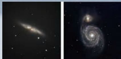
▲口径101cm望遠鏡とカメラを使い、 長時間露光で撮影したスターバースト 銀河(左)と子持ち銀河(右)
