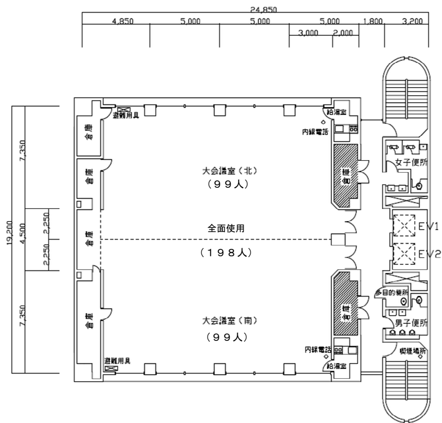
5階平面図
