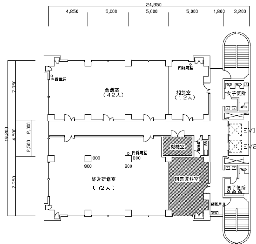
3階平面図
