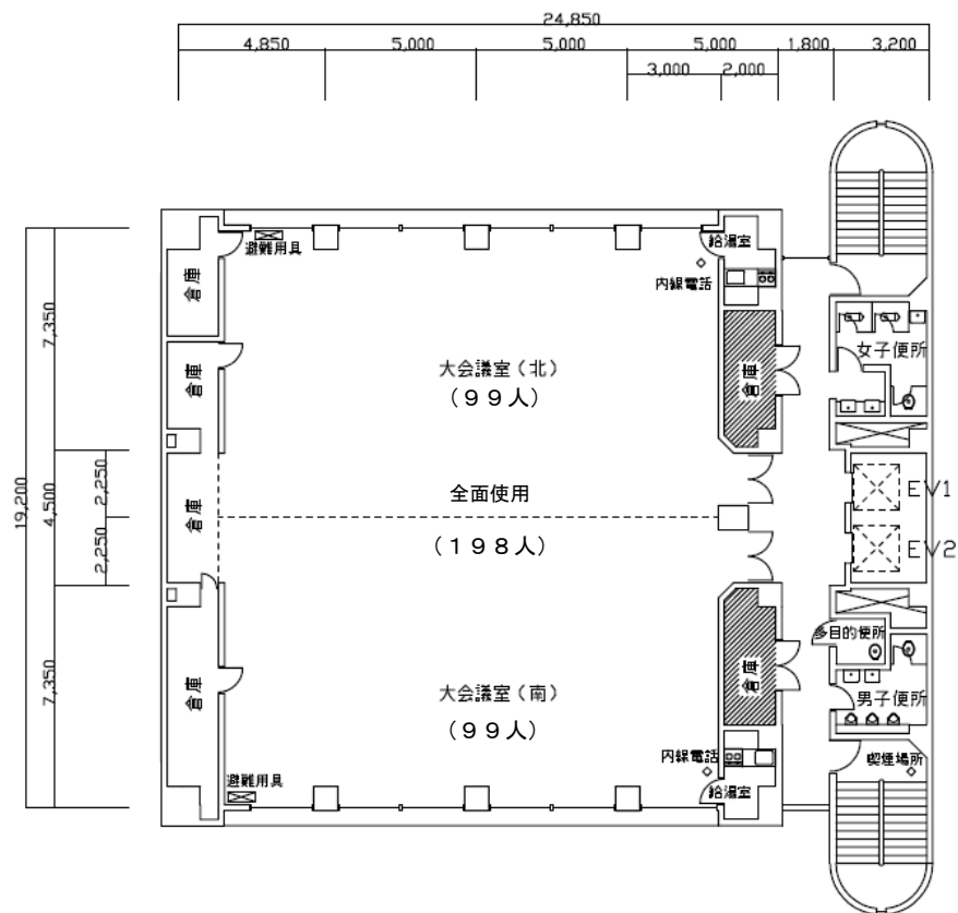
5階平面図
